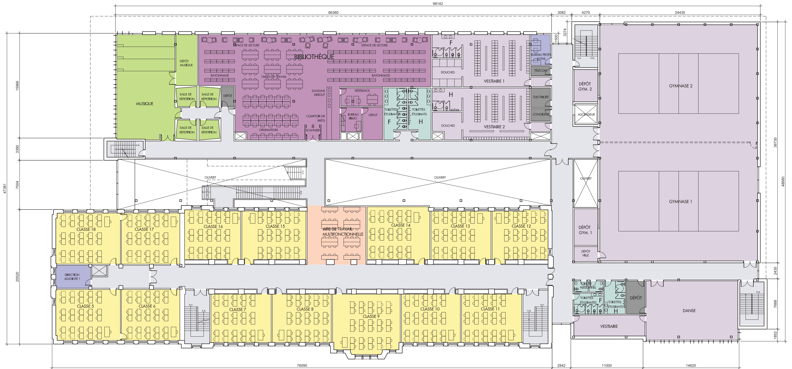
2ième ÉTAGE 1:300 21 JUIN 2011
